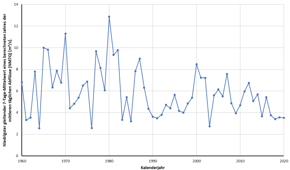
Abbildung 6: Ganglinie des jährlichen NM7Q am Pegel Epinal (1960-2020)
