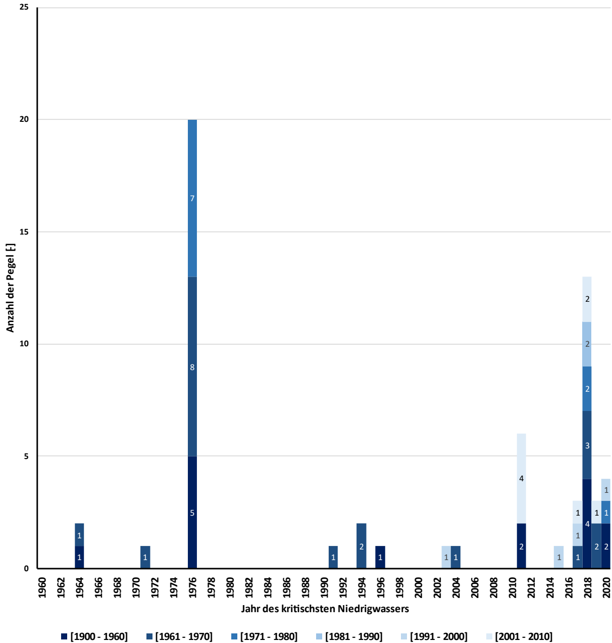
Abbildung 16: Jährliche Anzahl von Pegeln, die das Kriterium der maximalen Anzahl von Niedrigwassertagen erfüllen (1960-2020), mit Verteilung der jährlichen Anzahl nach Altersklassen
