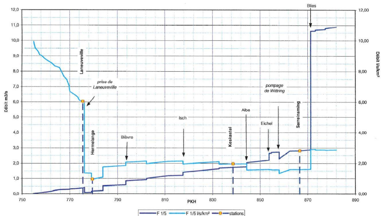
Abbildung 24: Entwicklung des monatlichen Mindestabflusses bei einer Wiederkehrzeit von T = 5 Jahren für die Saar (Quelle = Verzeichnis der Niedrigwasserabflüsse des Rhein-Maas-Einzugsgebiets – 2000)
