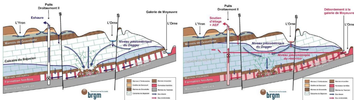
Abbildung 25: Prinzip der oberflächennahen Grundwasserführung der Orne bei Betrieb der Eisenminen Lothringens (links) und nach deren Stilllegung (rechts).
