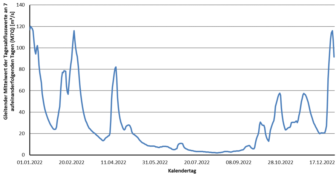
Abbildung 5: M7Q-Ganglinie am Pegel Epinal 2022
